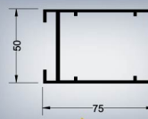
PV75 Porteur à feuillure
